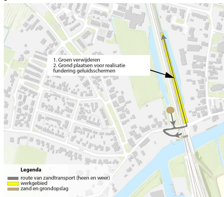
Figuur 1. Plattegrond werkzaamheden
